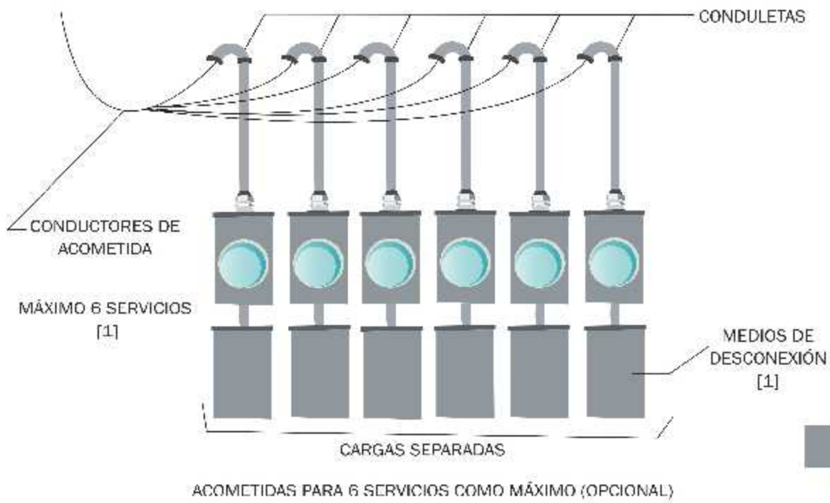
FIGURA #18 SERVICIOS CON ACOMETIDAS INDIVIDUALES
