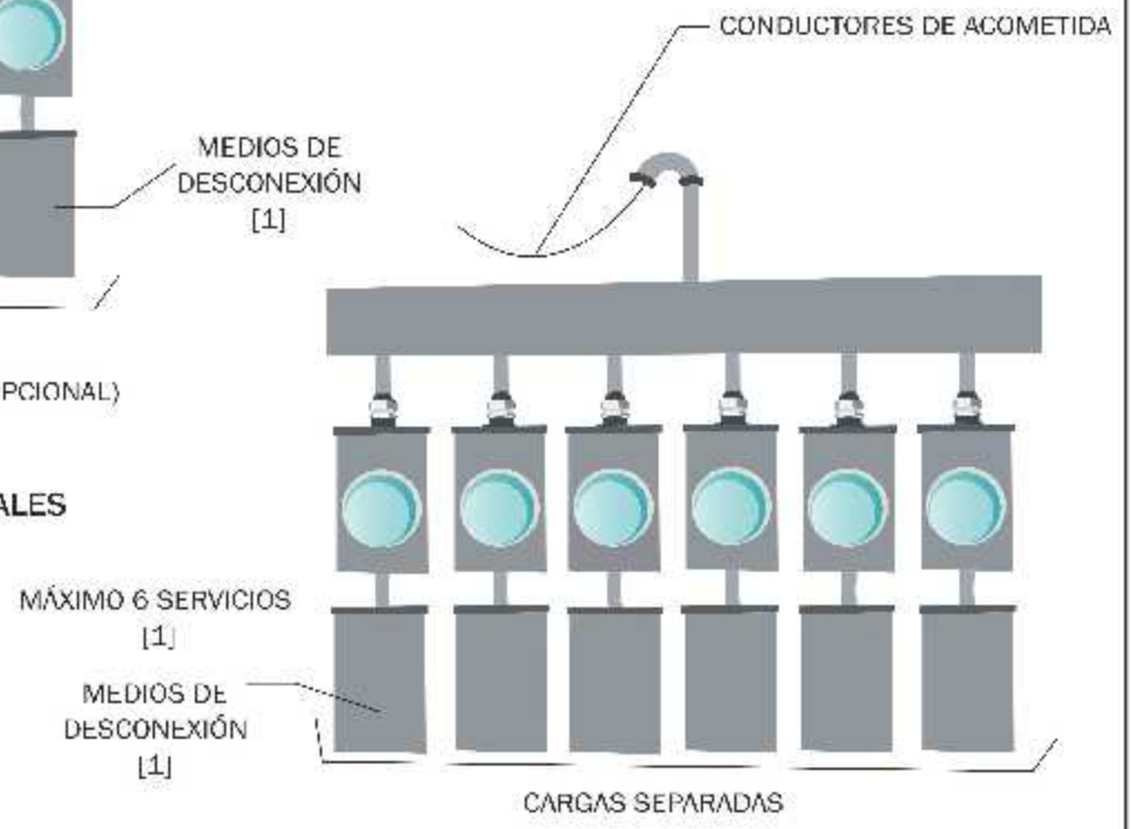
FIGURA #19 SERVICIOS CON ACOMETIDA ÚNICA ACOMETIDAS PARA 6 SERVICIOS MÁXIMO
