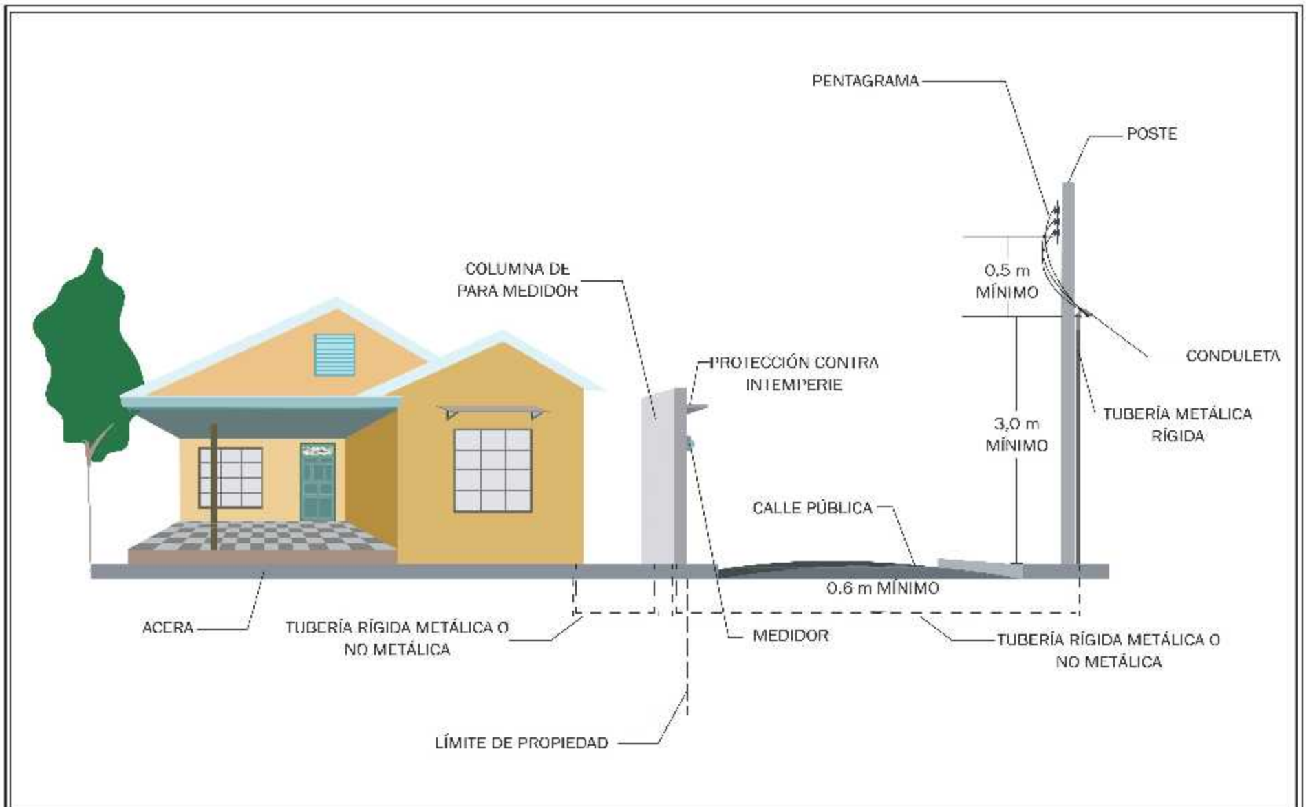
FIGURA #6 ACOMETIDA SUBTERRÁNEA DE BAJA TENSIÓN CON COLUMNA DE CONCRETO PARA MEDIDOR (PASO DE CALLE)
