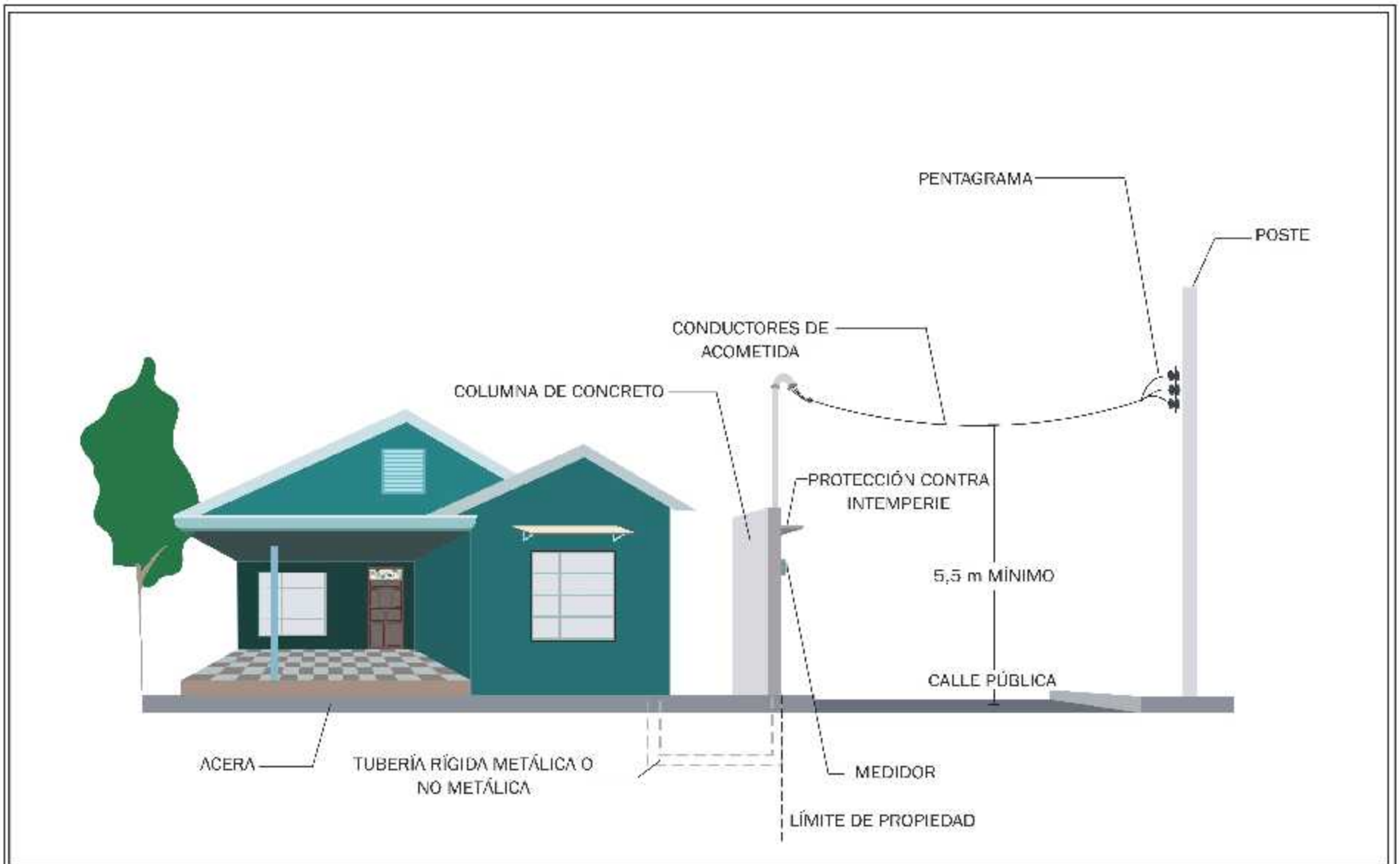
FIGURA #5 UBICACIÓN DEL EQUIPO DE MEDICIÓN EN MURO PEDESTAL (ENTRADA SUBTERRÁNEA)
