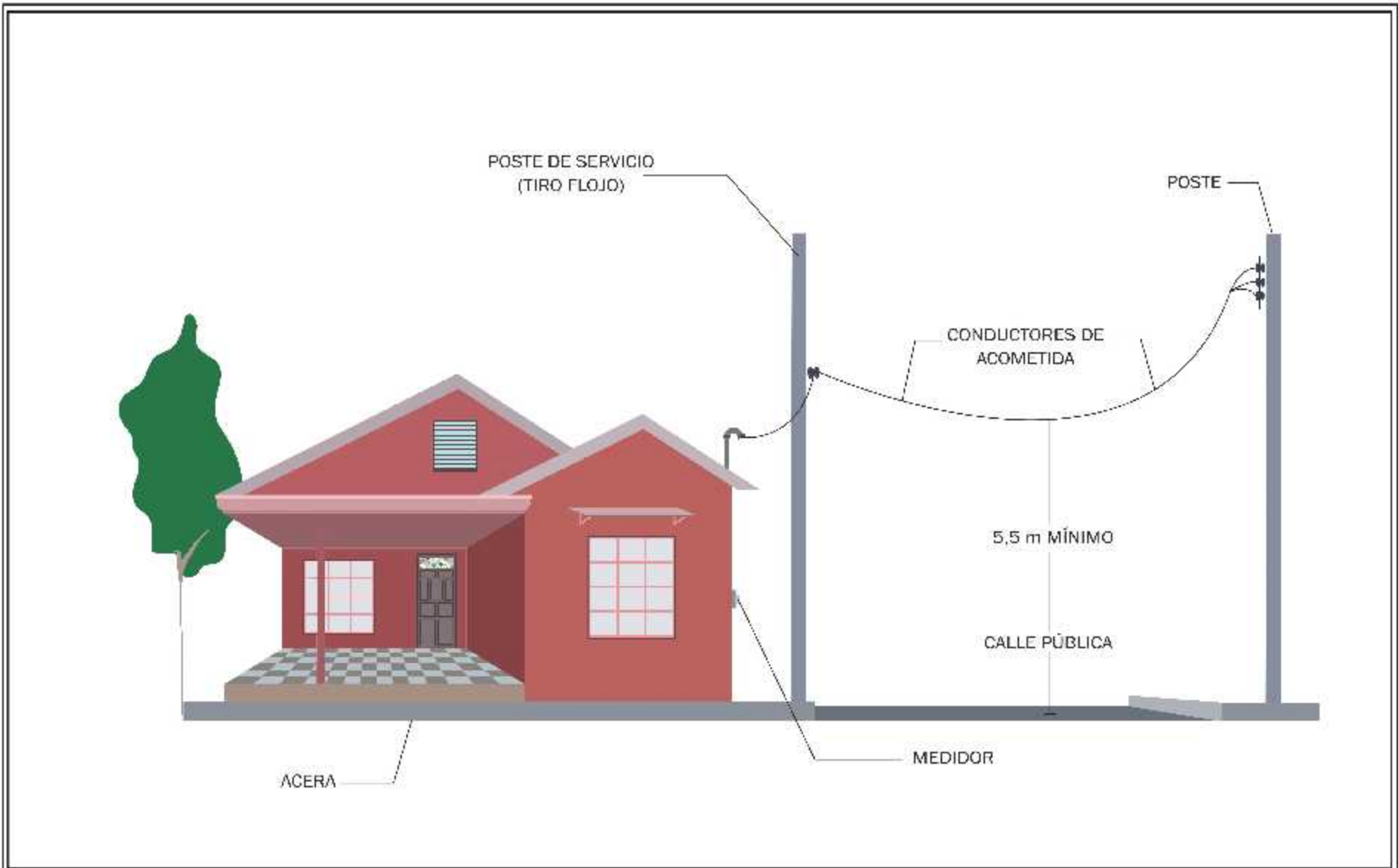
FIGURA #4 ALTURA PARA ACOMETIDA AÉREA A BAJA TENSIÓN CON POSTE DE SERVICIO (TIRO FLOJO)
