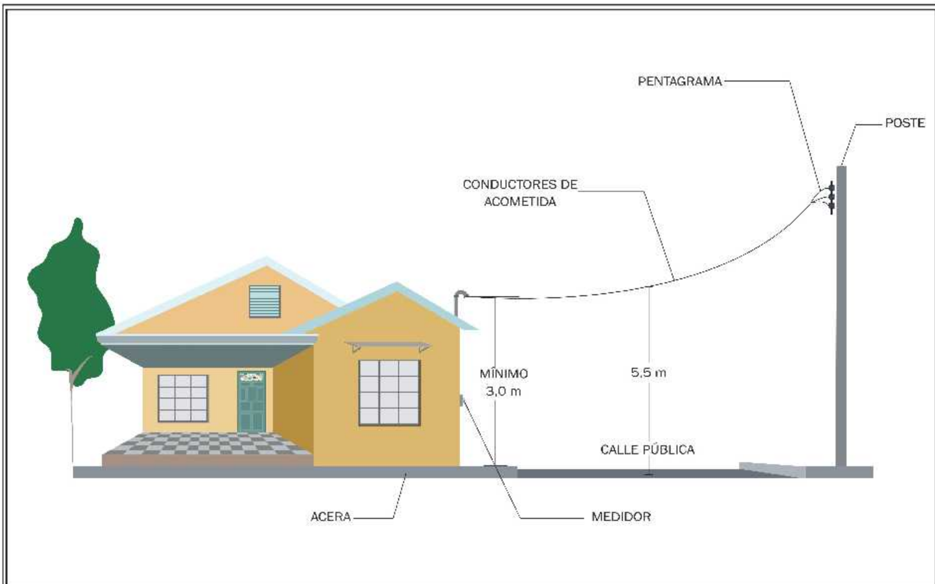
FIGURA #3 SEPARACIONES MÍNIMAS PARA CONDUCTORES DE ACOMETIDAS AÉREAS CON RESPECTO AL CENTRO DE LA CALLE PÚBLICA
