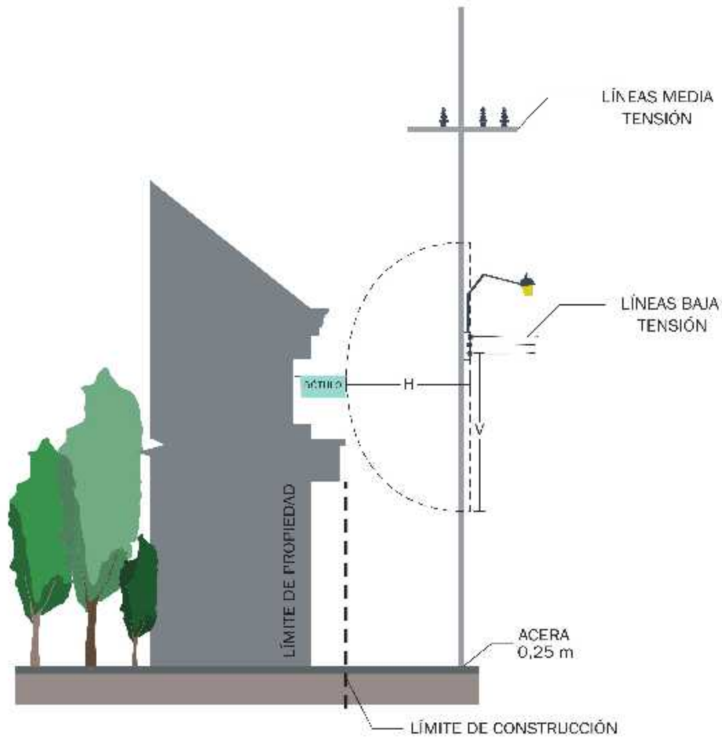
FIGURA #29 DISTANCIAS MÍNIMAS ENTRE CONDUCTORES DE DISTRIBUCIÓN Y EDIFICIOS (BAJA TENSIÓN)
