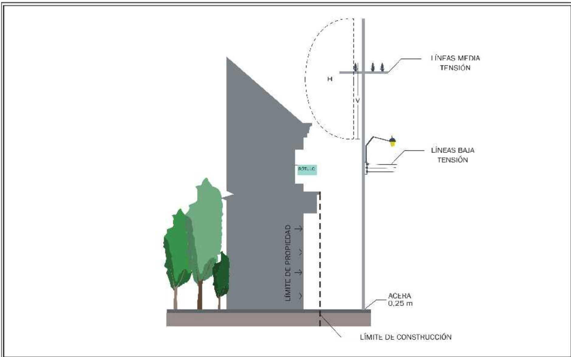
FIGURA #28 DISTANCIAS MÍNIMAS ENTRE CONDUCTORES DE DISTRIBUCIÓN Y EDIFICIOS (MEDIA TENSIÓN)
