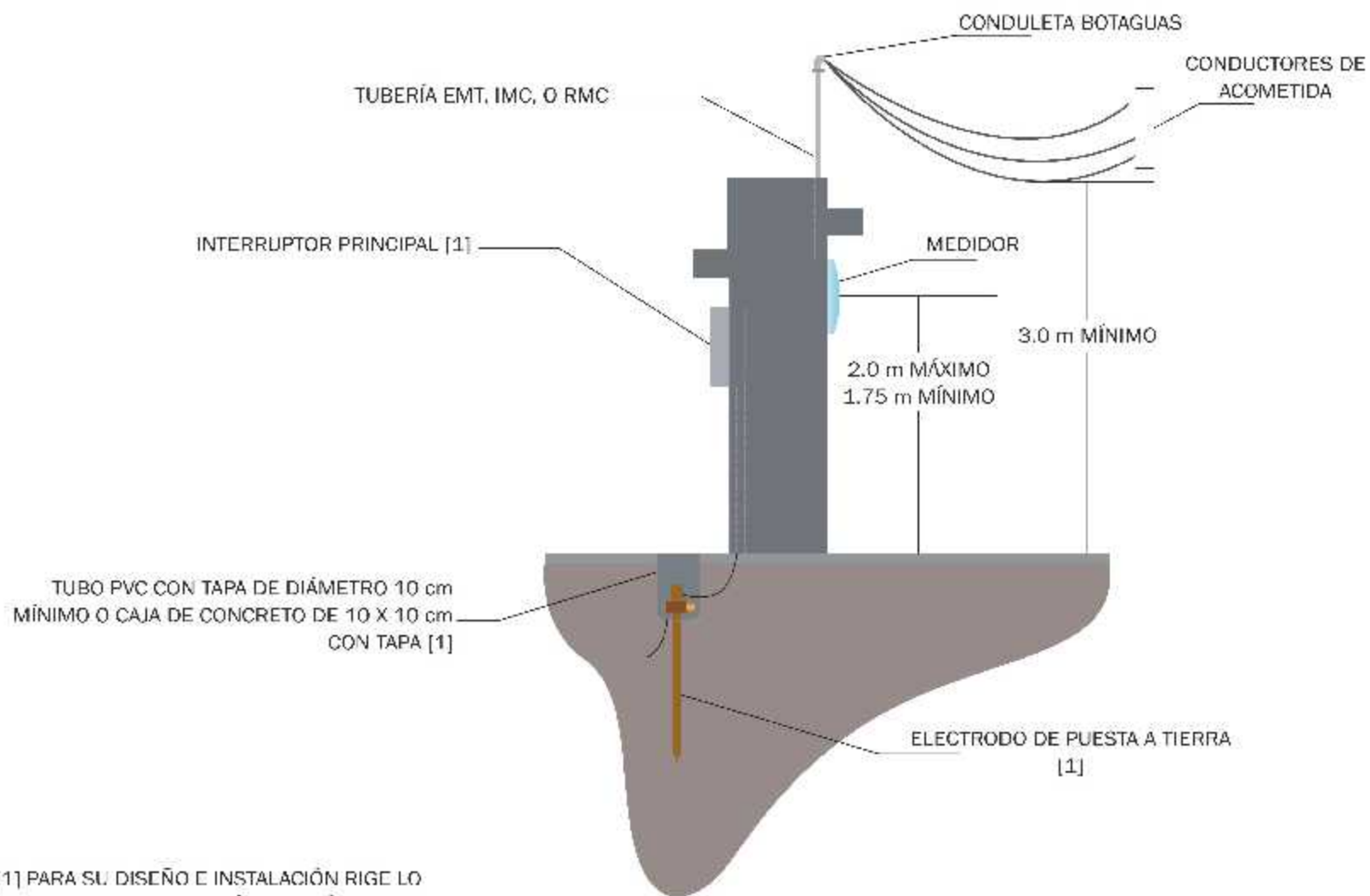
FIGURA #27 UBICACIÓN DEL ELECTRODO DEL SISTEMA PUESTA A TIERRA
