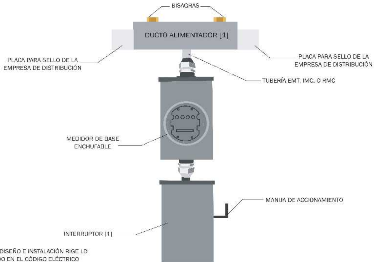
FIGURA #26 DIAGRAMA DE CONEXIÓN MECÁNICA PARA MEDIDORES EN EDIFICIOS DE OCUPACIÓN MÚLTIPLE
