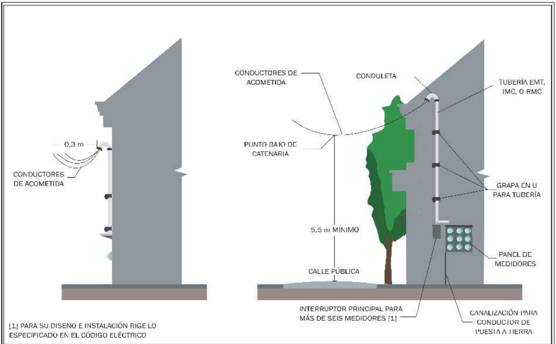
FIGURA #25 UBICACIÓN DE PANELES PARA MEDIDORES EN PARED EXTERIOR CON MEDIO DE DESCONEXIÓN PRINCIPAL
