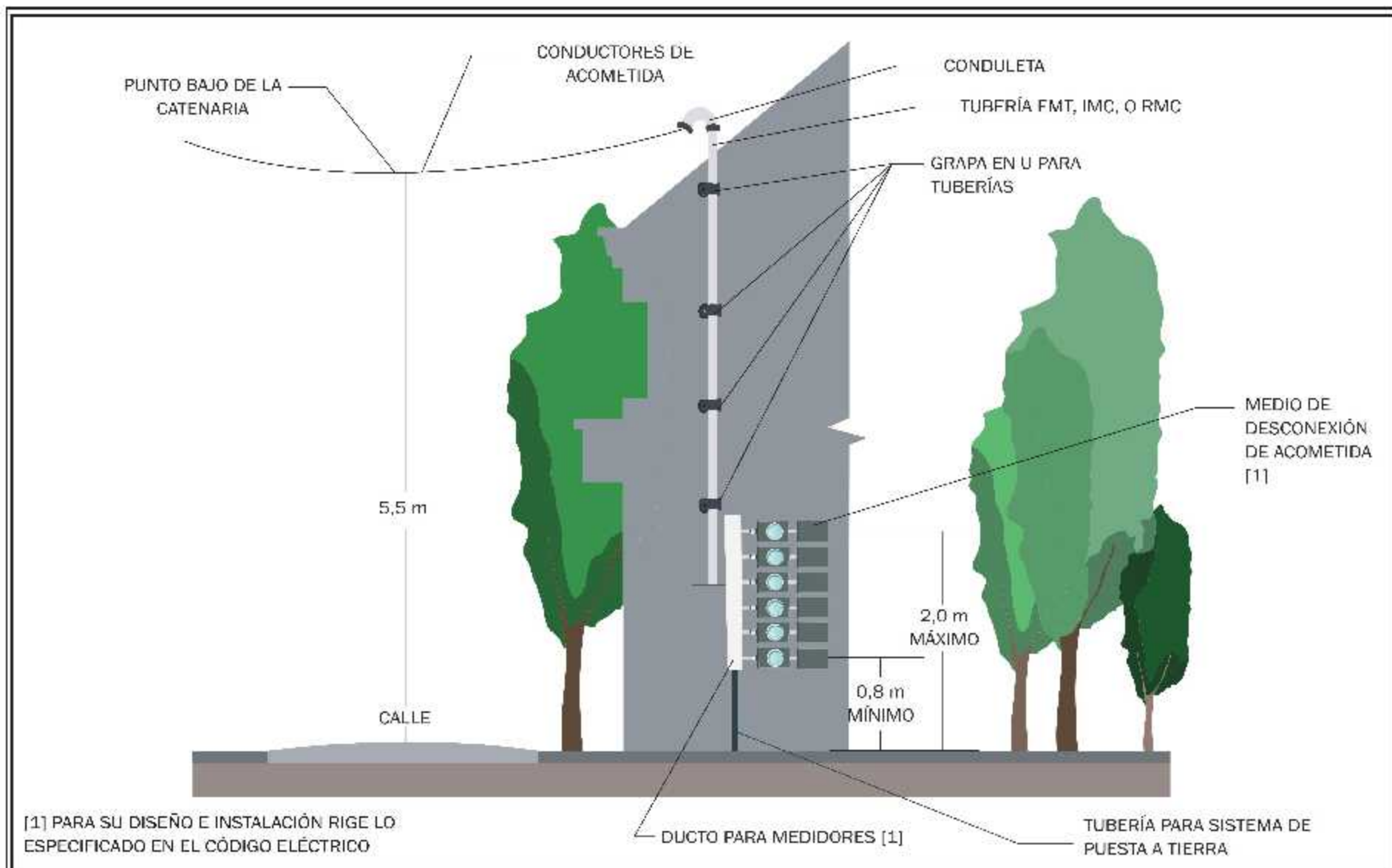
FIGURA #22 UBICACIÓN DE MEDIDORES MÚLTIPLES EN DUCTO VERTICAL CON ACOMETIDA GENERAL
