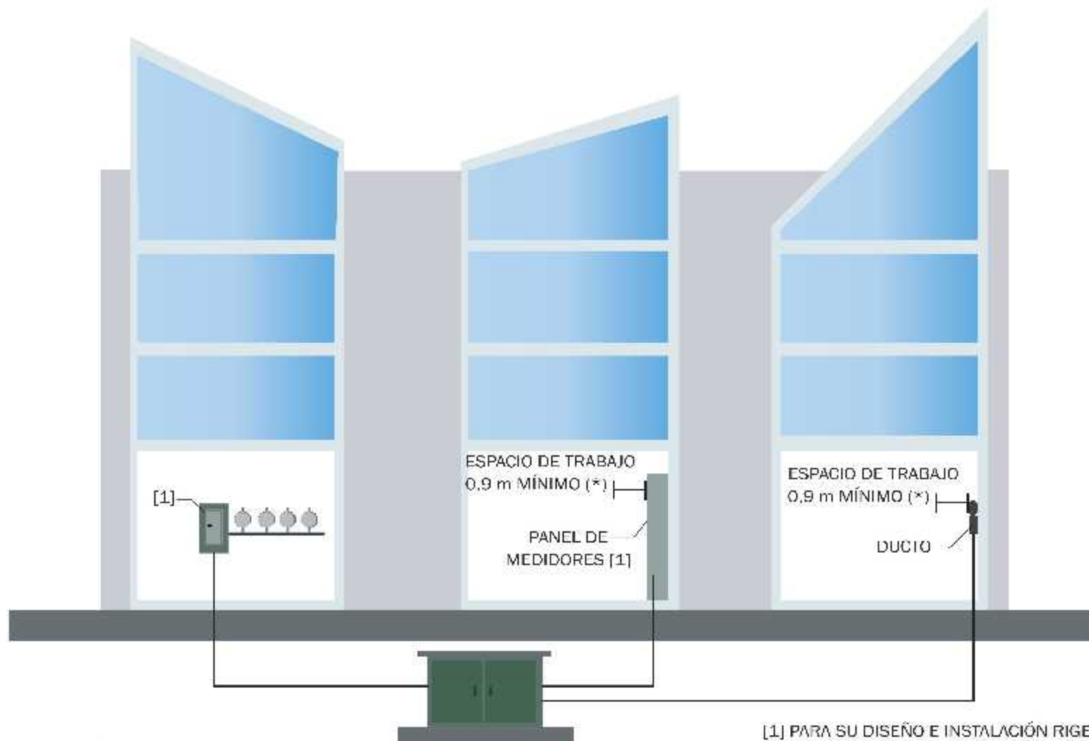
FIGURA #20 DISTRIBUCIÓN CON TRANSFORMADORES DE PEDESTAL EN CENTRO COMERCIALES CON DUCTOS MÚLTIPLES DE MEDIDORES
