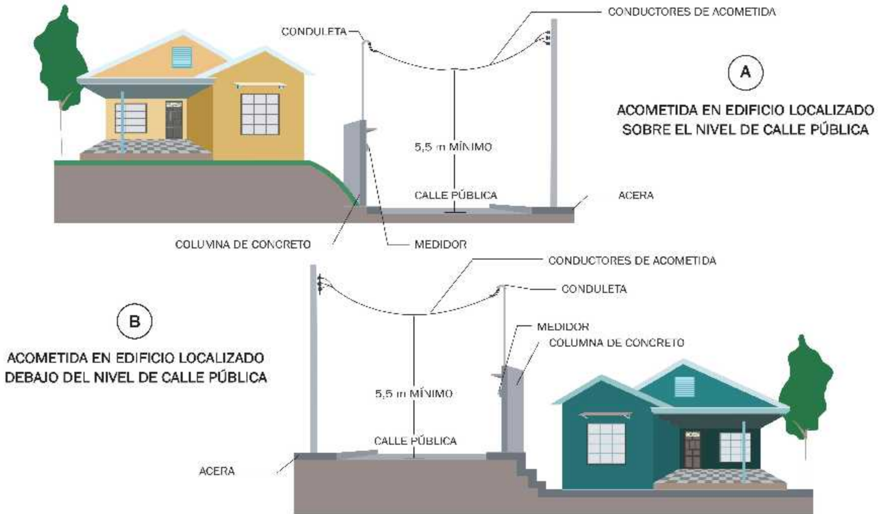
FIGURA #17 ACOMETIDAS EN EDIFICIOS LOCALIZADOS SOBRE O DEBAJO DEL NIVEL DE CALLE PÚBLICA
