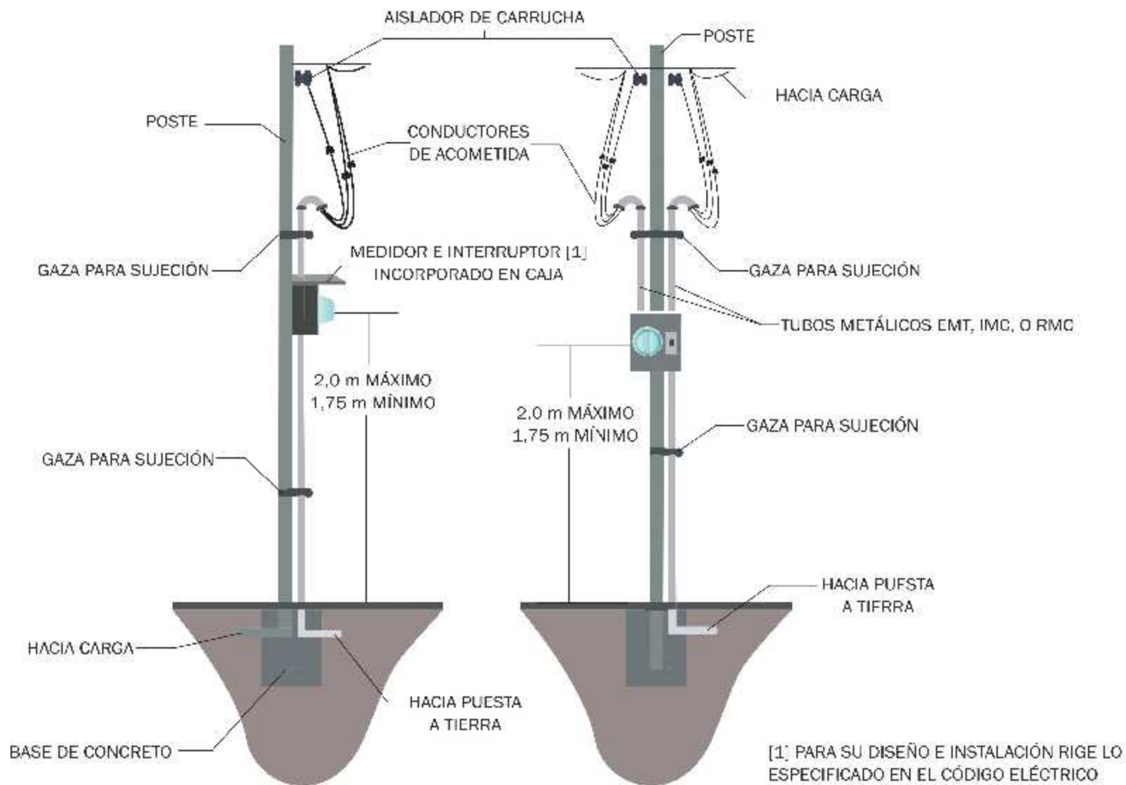
FIGURA #16 INSTALACIÓN DE ACOMETIDA EN POSTE CON INTERRUPTOR [1] INCORPORADO EN CAJA DE MEDIDOR
