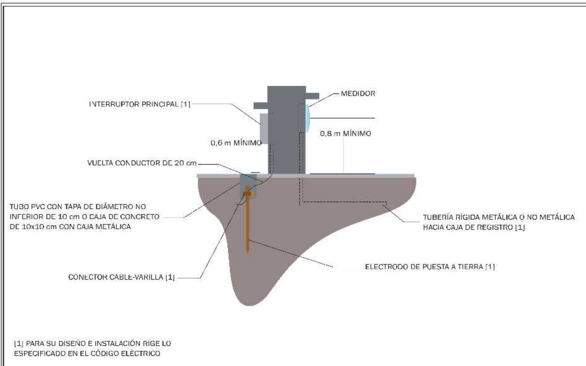
FIGURA #14 UBICACIÓN DE EQUIPO DE ACOMETIDA SUBTERRÁNEA CON MEDIDOR UBICADO HACIA LA CALLE DE ACCESO PÚBLICO
