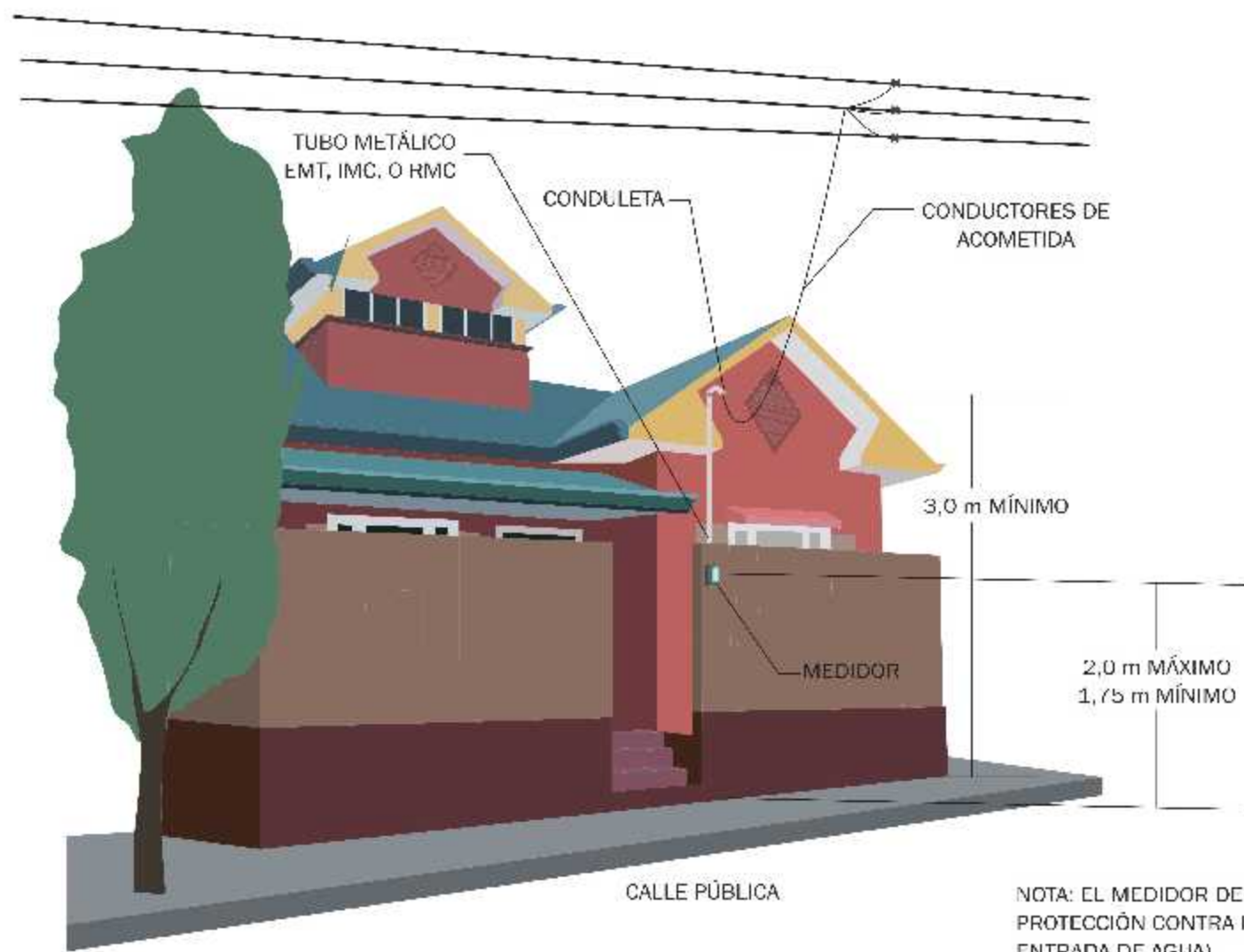
FIGURA #13 ACOMETIDA EN EDIFICACIÓN CON TAPIA (MEDIDOR EN TAPIA FRENTE A CALLE PÚBLICA)
