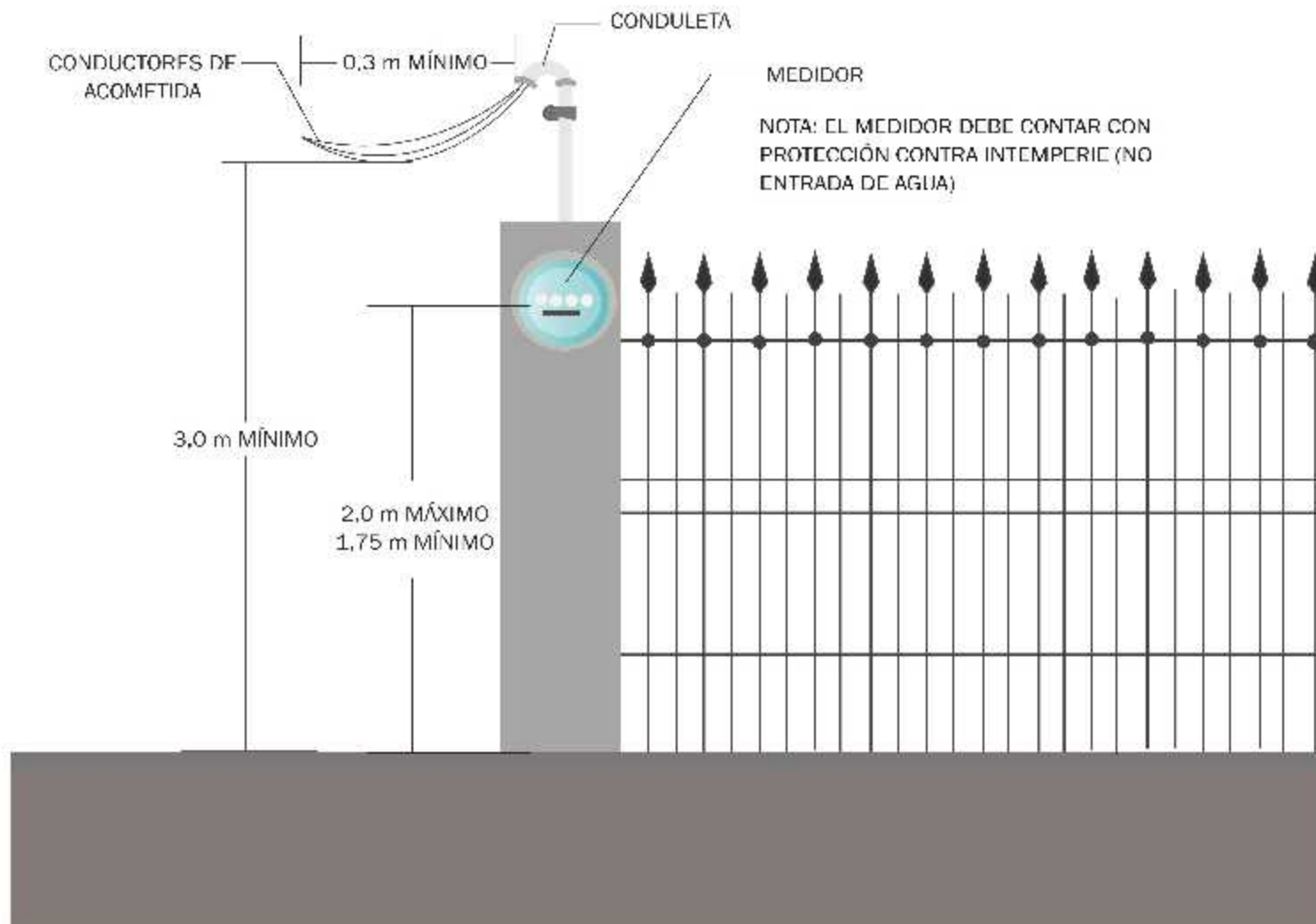
FIGURA #11 ACOMETIDA EN EDIFICACIÓN SIN MURO AL FRENTE (MEDIDOR EN LÍMITE DE PROPIEDAD)
