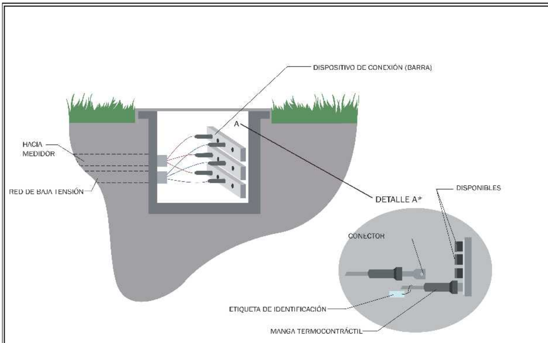
FIGURA #10 DISPOSITIVOS DE CONEXIÓN EN ACOMETIDAS SUBTERRÁNEAS DE BAJA TENSIÓN
